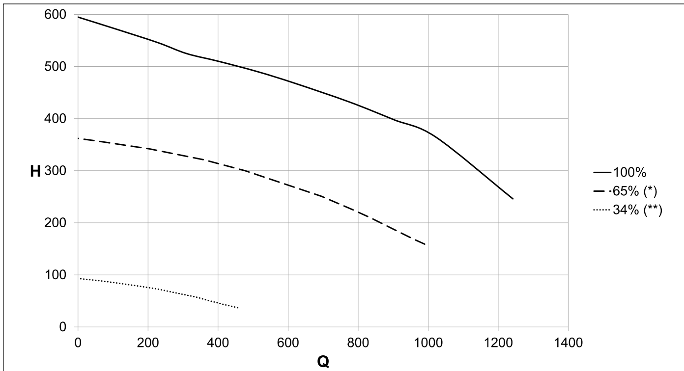
Fig. 28 Presiune disponibilă KC-KR-KRB 32
