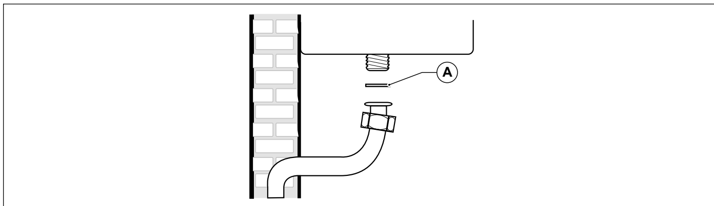
Fig. 22 Racordare la rețeaua de gaz
