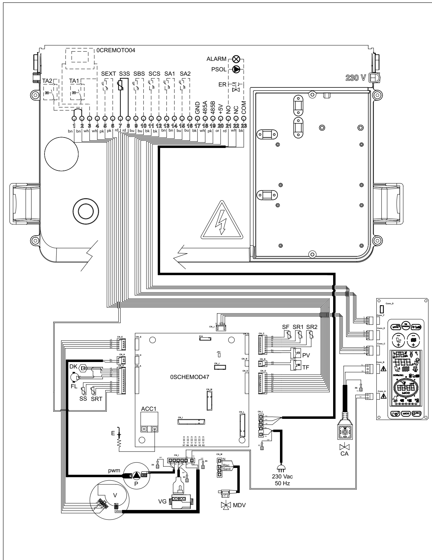
Fig. 29 Schema electrică KC
